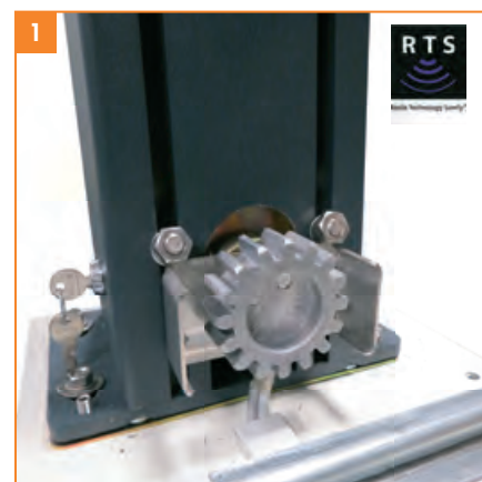
Moteur intégré dans le poteau de guidage
