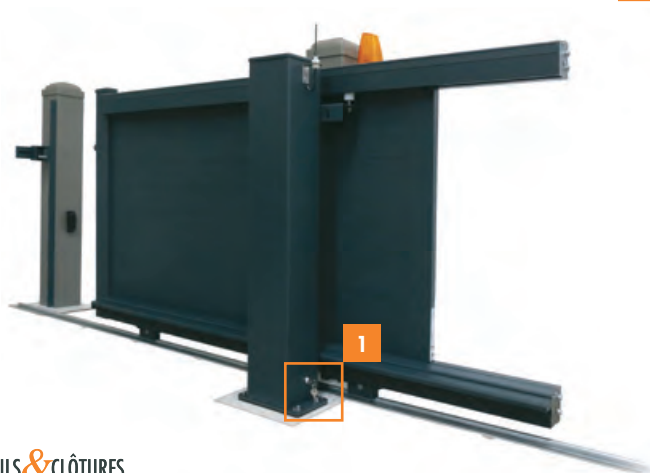
Moteur intégré dans le poteau de guidage
